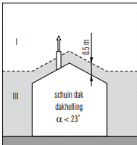
Afbeelding 8.4: Minimale afvoerhoogte bij bestaande afvoer (bron: website Schone Lucht Akkoord).
