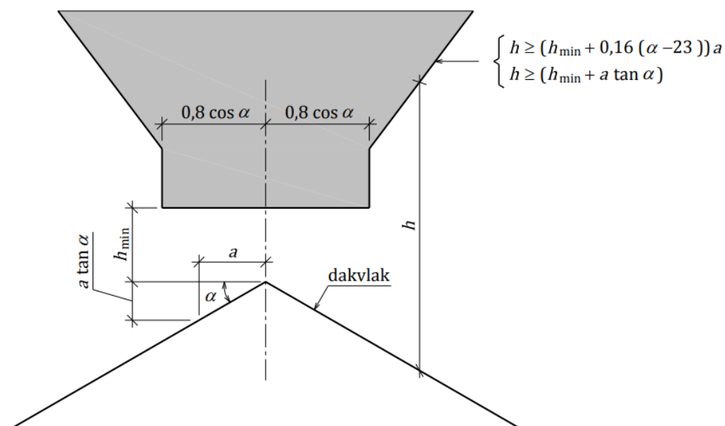
Figuur 3 —Uitmondingshoogten en vrij uitmondingsgebied
