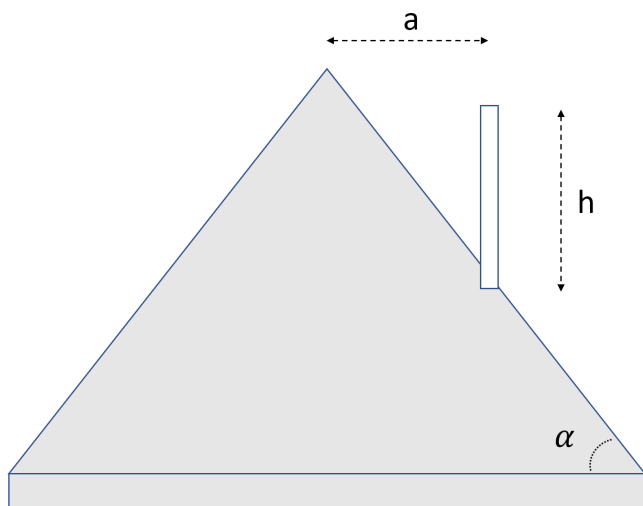
Afbeelding 8.5: Weergave van de drie variabelen als gebruikt in paragraaf 5.2.3 in NEN 8757.
