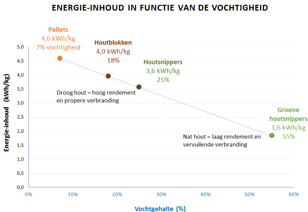
Afbeelding 3.3: Energie-inhoud van houtachtige brandstoffen in relatie tot het vochtgehalte (bron: www.ode.be )
